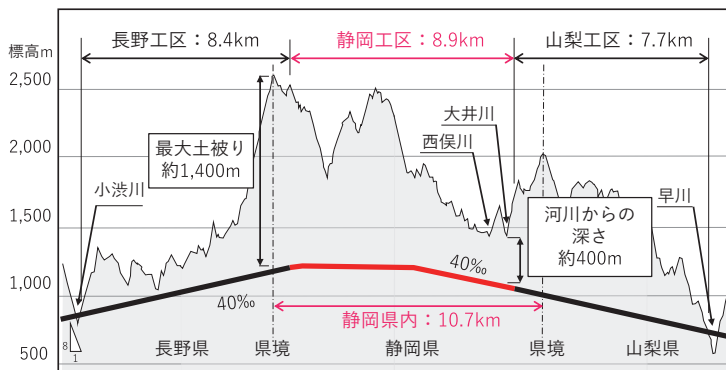
図3.トンネルの縦断面図
