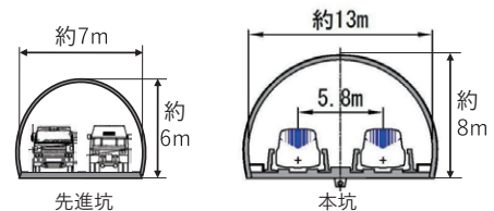
図7.トンネル断面図
